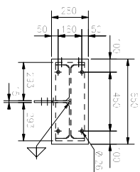
DETAIL POS. - 5 -
