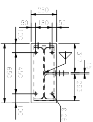
DETAIL POS. - 6 -
