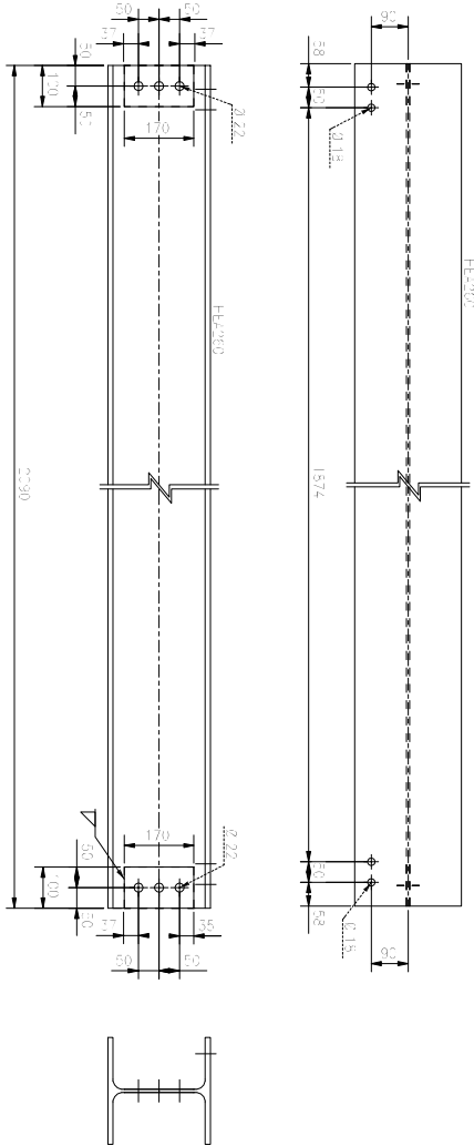
DETAIL POS. 27
