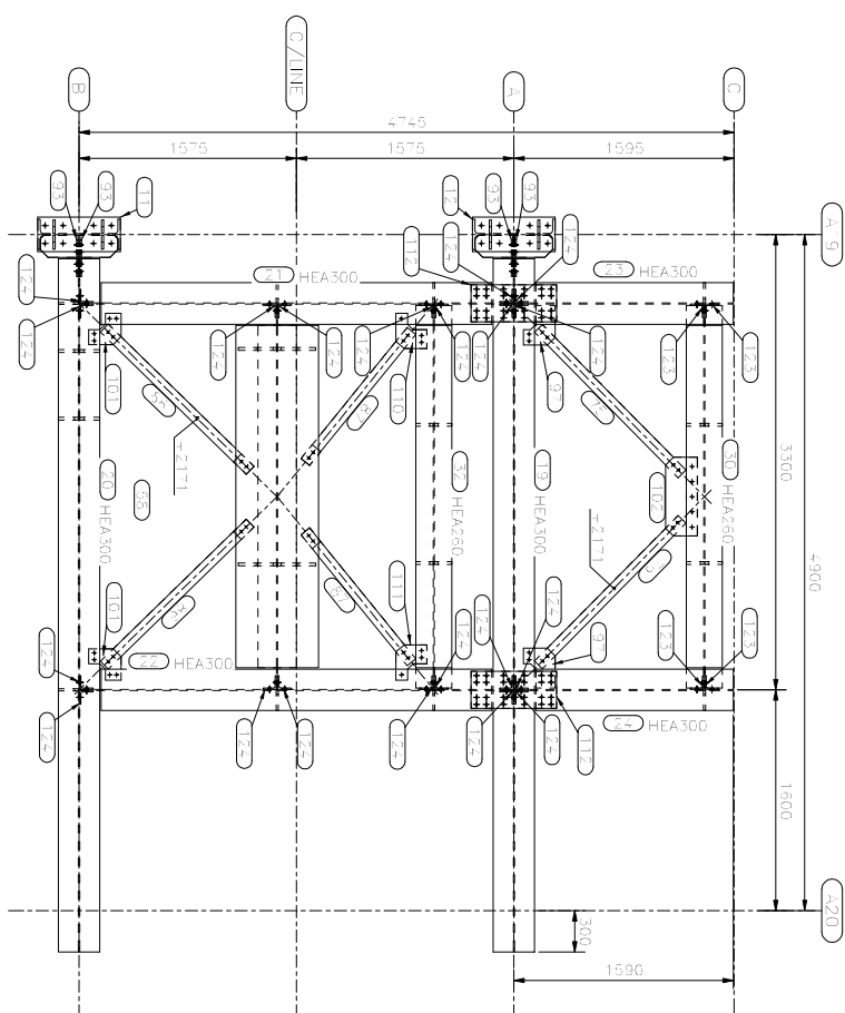
Plan +2195
