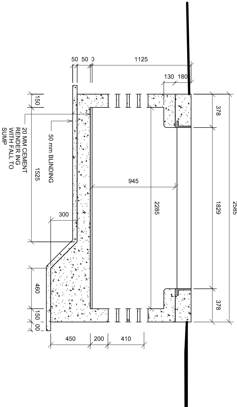
ELEVATION - A
