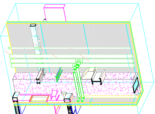
5 | VIEW 5 SCALE: 1/8"
