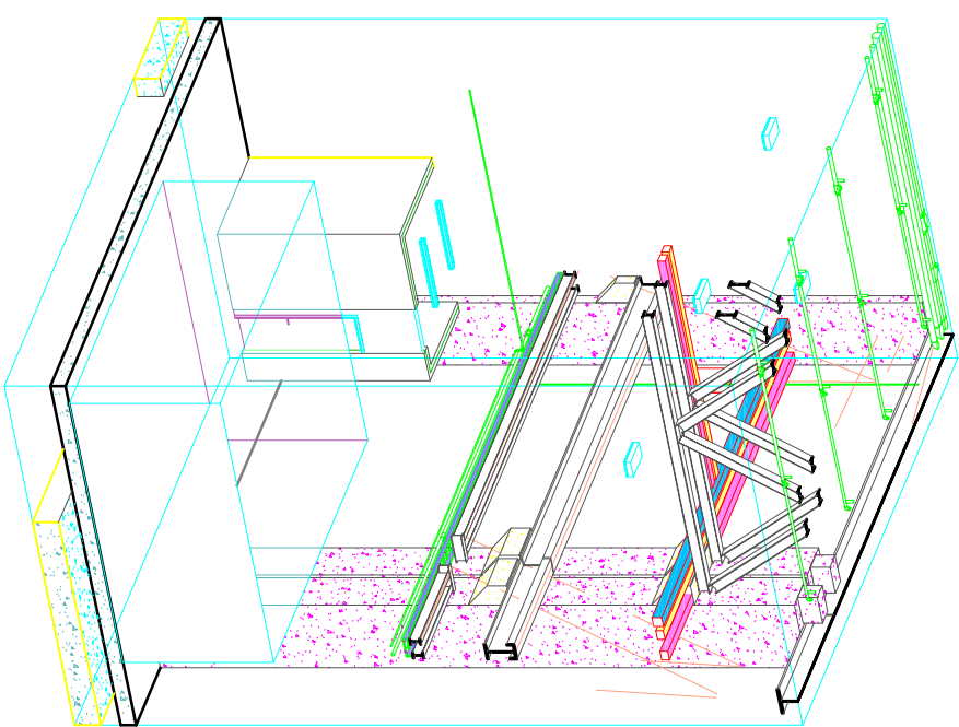
4 | VIEW 4 SCALE: 1/8"
